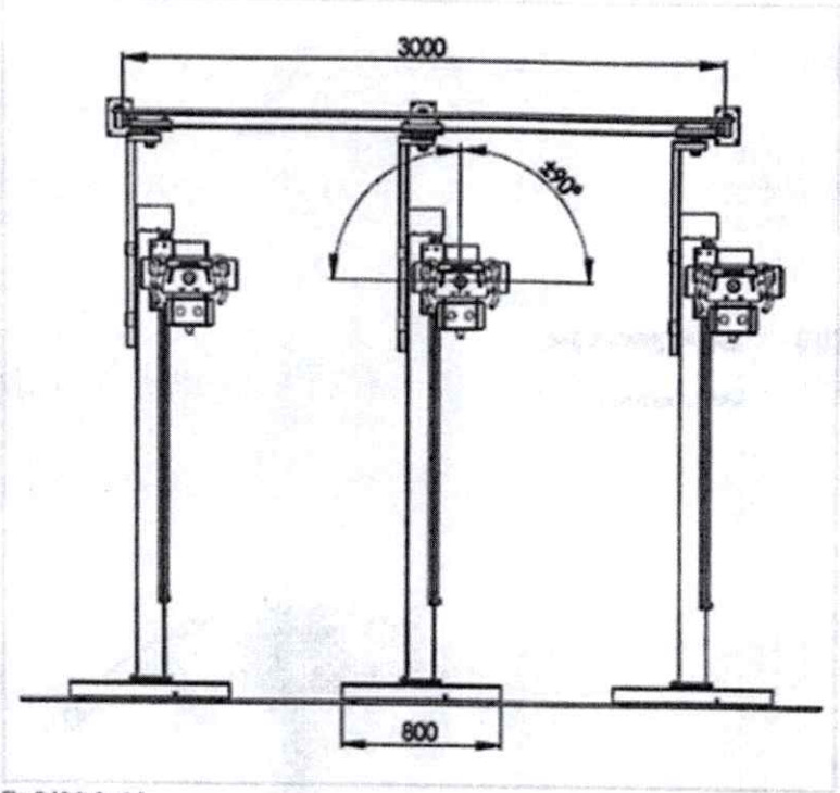
Fig. 2: Vista frontal
