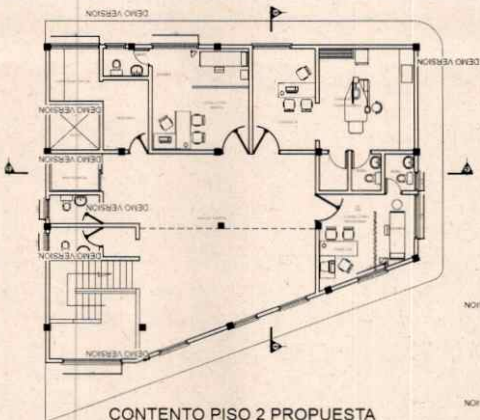
Planta Propuesta de Piso 2
